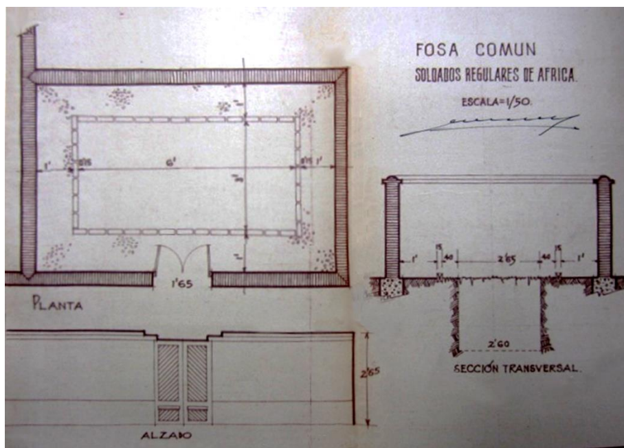
Plano del cerramiento y fosa común de los restos de los regulares de África enterrados fuera del recinto del cementerio
